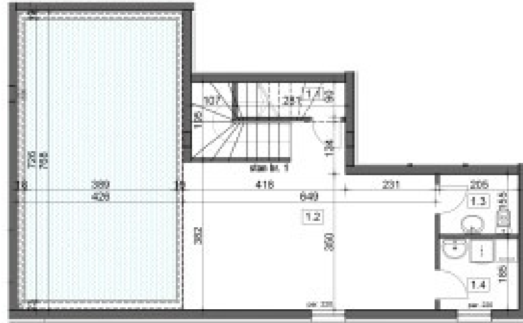
OSNOVA PODRUMA
