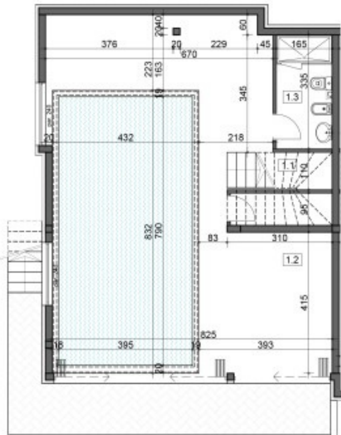
OSNOVA PODRUMA
