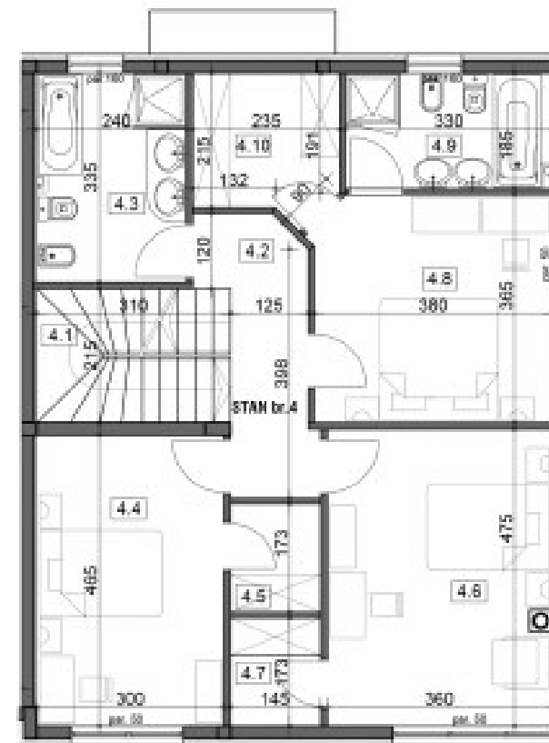
OSNOVA 1. SPRATA
