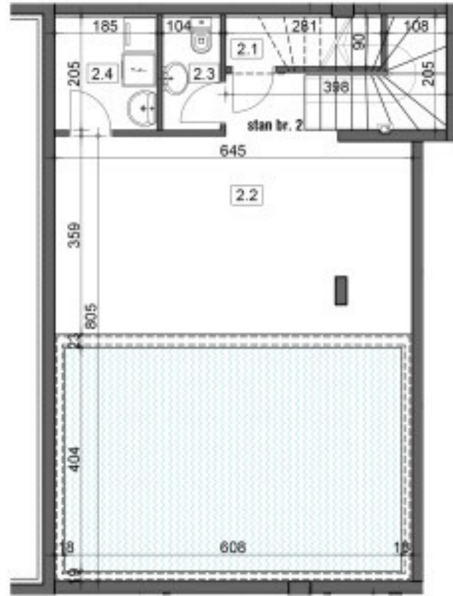
OSNOVA PODRUMA
