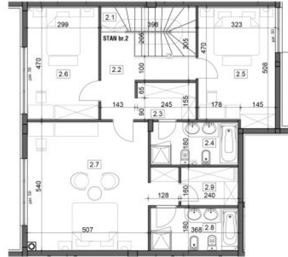
OSNOVA 1. SPRATA
