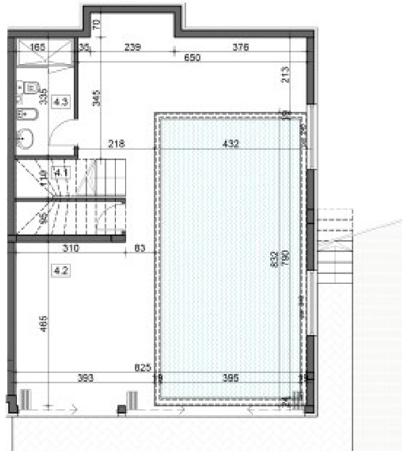
OSNOVA PODRUMA
