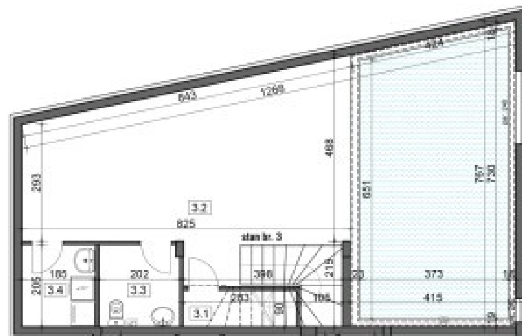
OSNOVA PODRUMA
