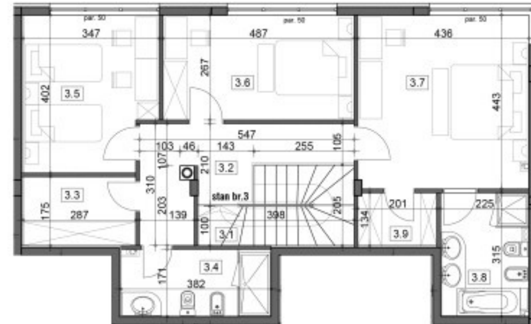
OSNOVA 1. SPRATA
