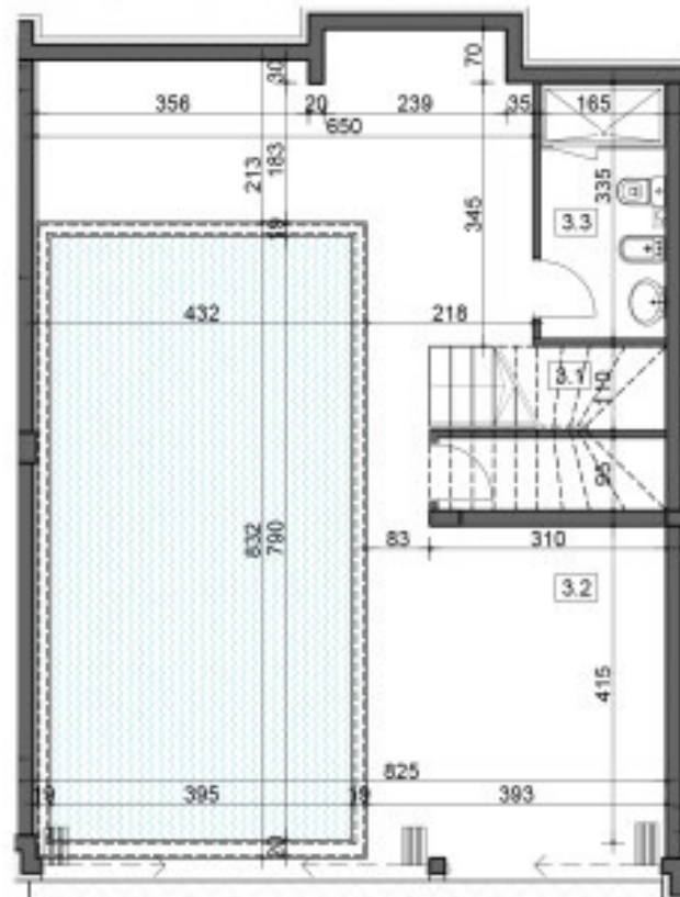
OSNOVA PODRUMA
