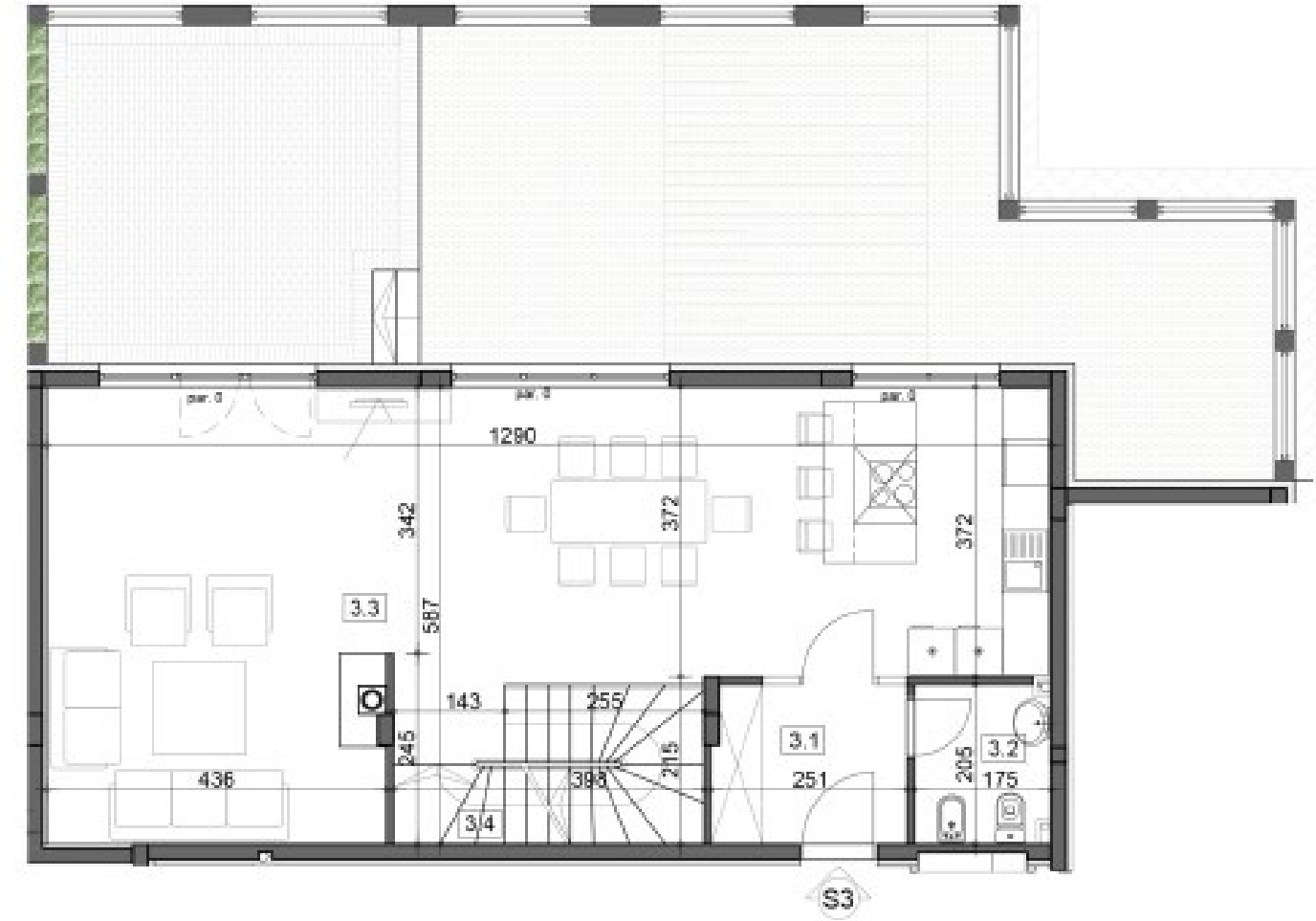
OSNOVA PRIZEMLJA
