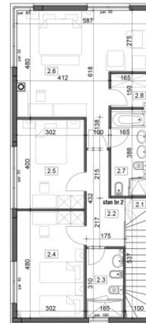
OSNOVA 1. SPRATA
