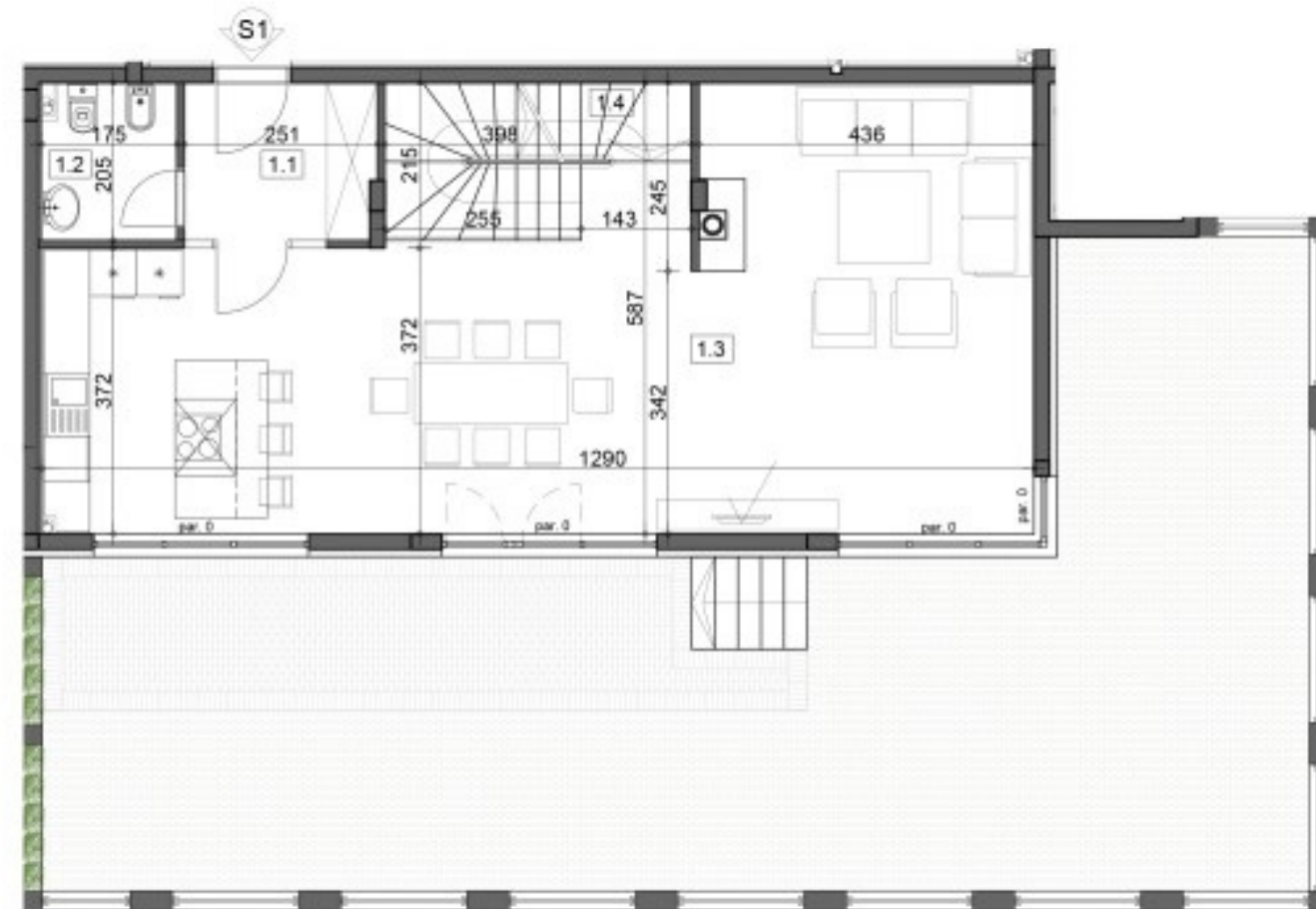
OSNOVA PRIZEMLJA
