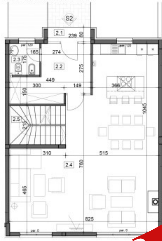
OSNOVA PRIZEMLJA
