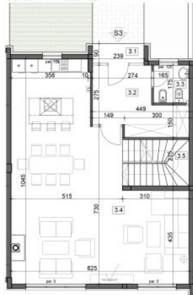
OSNOVA PRIZEMLJA
