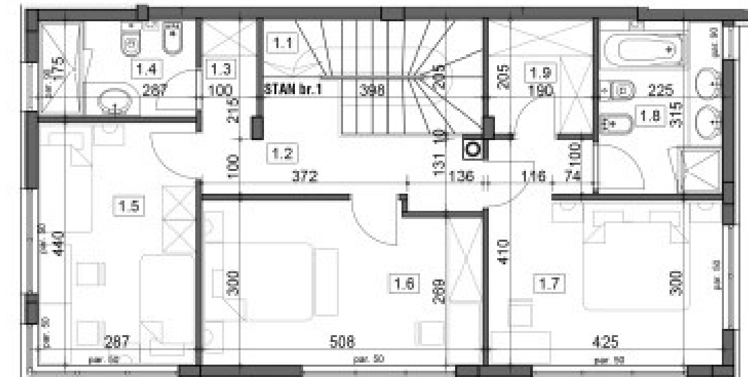
OSNOVA 1. SPRATA
