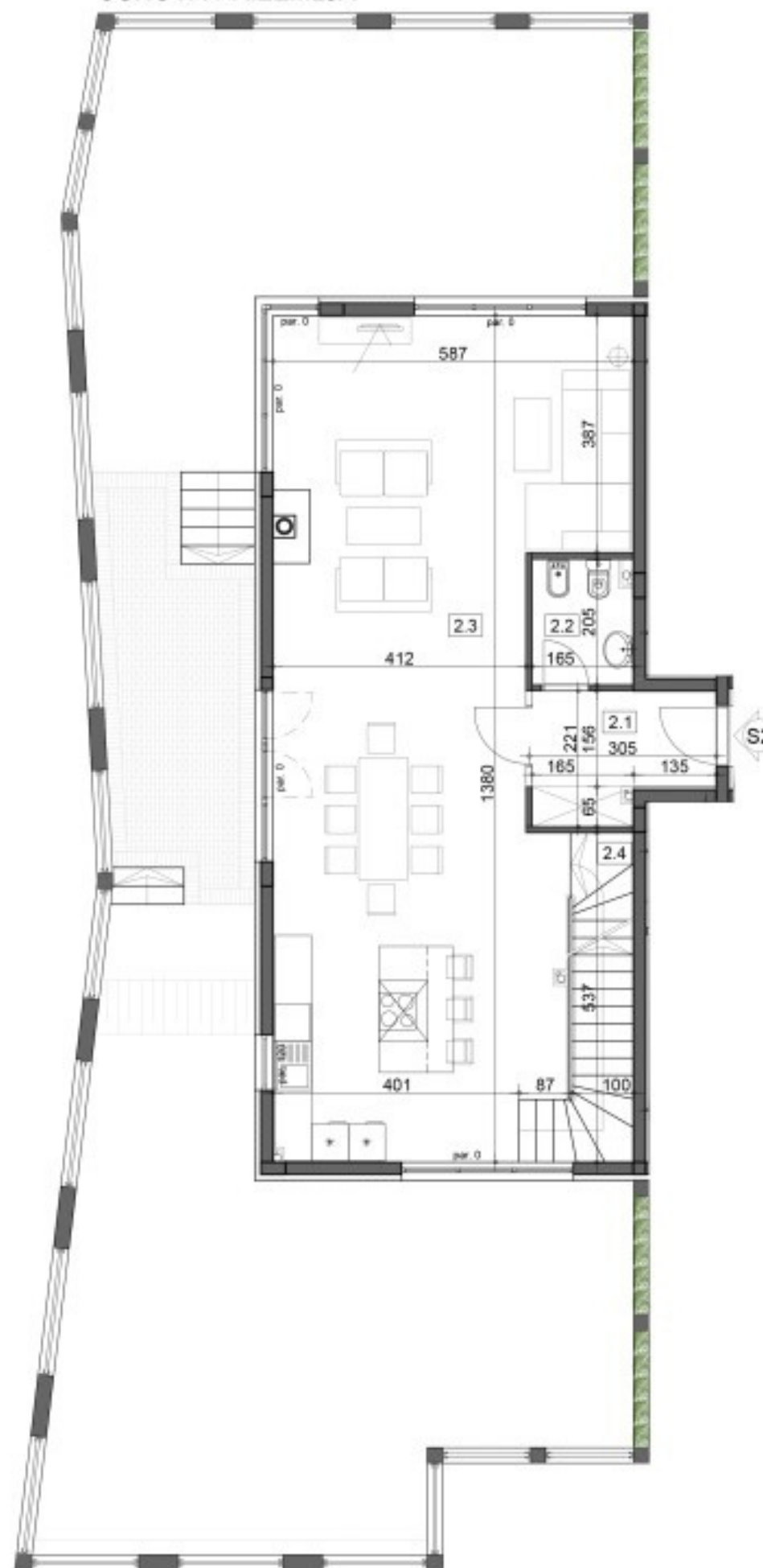
OSNOVA PRIZEMLJA
